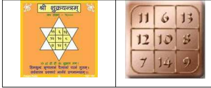
Venüs Yantra
